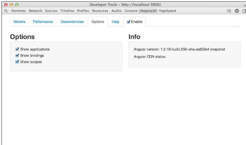
Batarang options
