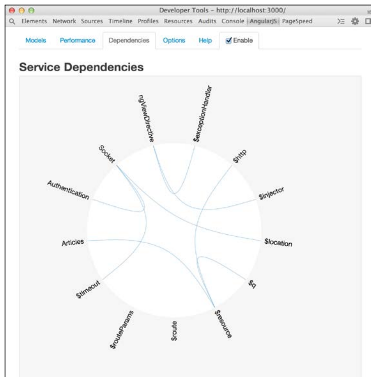
Batarang dependencies
