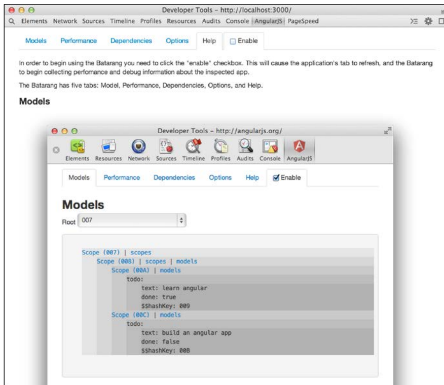
Batarang Tool
